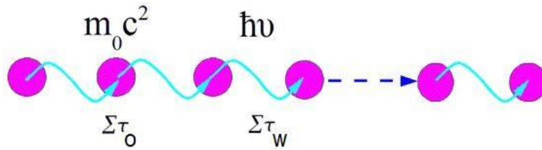
Рис. 1. Условная кинематическая схема дискретного движения микрообъектов. Заполненными кружками изображен объект в поочередном состоянии «объект» в абсолютной системе отсчета ФВ. Состояние «собственно» объект характеризуется параметром m_0 c^2 , а длительность пребывания в этом состоянии равна сумме элементарных временных актов \Sigma \tau_0 . Параметр \hbar \nu характеризует волновой процесс в ФВ. \Sigma \tau_w определяет длительность волнового процесса в виде суммы элементарных временных актов.
